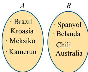
Gambar 2.2 Himpunan A dan Himpunan B
