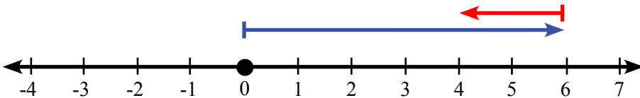
Gambar 1.8 Pengurangan 6 - 2 pada garis bilangan
