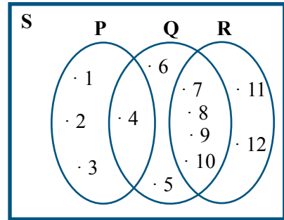
Gambar 2.22 Diagram Venn a dan b
