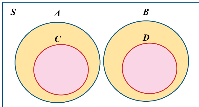
Gambar 2.8 Diagram Venn dari Masalah 2.5
