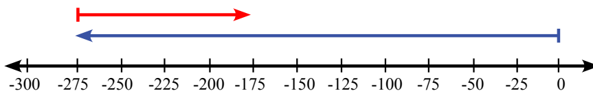
Gambar 1.13 Lawan (negatif) dari 275 - 100
